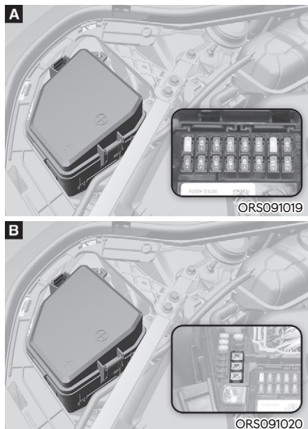
㉠: 블레이드 타입, ㉡: 카트리지 타입
