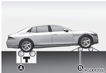
Ⓐ: 롤 테스터, Ⓑ: 간이식 프리 롤 장치
