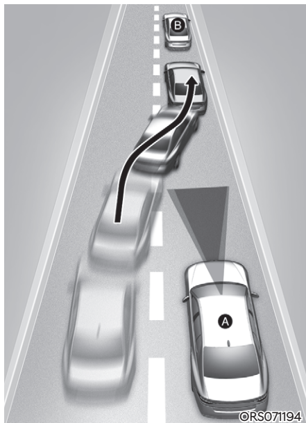
Ⓐ: 자차, Ⓑ: 차로변경 차량
