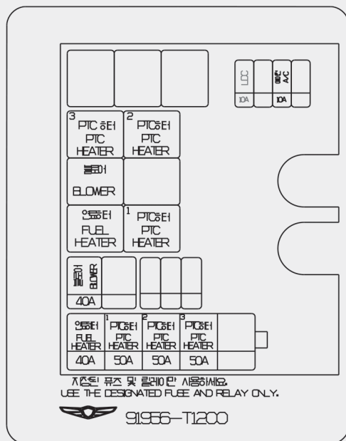
엔진룸 (퓨즈/릴레이 박스) 라벨 (동승석 쪽)
